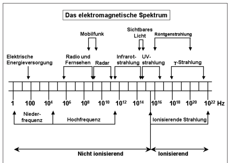
ABBILDUNG 1: Das elektromagnetische Spektrum (modifiziert nach Repacholi, 1996). Das elektromagnetische Spektrum wird in Frequenzbereiche mit sehr unterschiedlichen Eigenschaften und biologischen Wirkungen unterteilt. Zu den statischen Feldern (0 Hertz) gehört z. B. das natürliche Erdmagnetfeld. Künstlich erzeugte statische Magnetfelder werden u. a. zur Kernspintomographie verwendet. Der Bereich der niederfrequenten Felder enthält u. a. elektrische oder magnetische Felder im extrem niedrigen Frequenzbereich von > 0 bis 300 Hertz. In diesem Frequenzbereich liegt z. B. der Wechselstrom mit 50 oder 60 Hertz. Hochfrequente elektromagnetische Felder (im Englischen auch als „Radiofrequency [RF] fields“ bezeichnet) haben Frequenzen zwischen 30 000 Hertz und 300 Giga-Hertz. Wie bei statischen oder niederfrequenten Feldern gilt die Energie dieser Felder i. G. zu UV-Licht und ionisierender Strahlung als zu schwach, um Moleküle zu ionisieren oder chemische Bindungen zu brechen und damit direkte DNS-Schädigungen hervorzurufen. RF-Felder werden für alle Arten von Informationsübertragung, also Radio (AM, FM), Fernsehen, Mobilfunk und Radar verwendet. Erst oberhalb dieses Hochfrequenzbereiches spricht man von Strahlung. Immer noch im nicht-ionisierenden Bereich (von \sim 10^{12} – 10^{17} Hertz) liegt die optische Strahlung, zu der Infrarot, sichtbares Licht und UV-Strahlung gehören. Im Frequenzbereich von > 10^{15} – 10^{22} liegt die ionisierende Strahlung (Röntgen- und Gamma-Strahlung).
